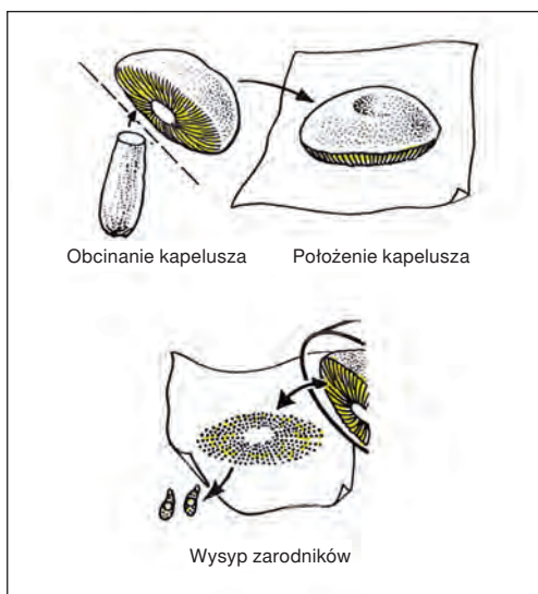
Ryc. 2. Pozyskiwanie zarodników
